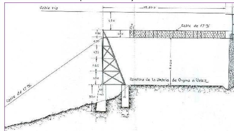
Fig. 5. Detalle de sección en cruzamiento de la línea con un vial. Fuente: proyecto constructivo.
